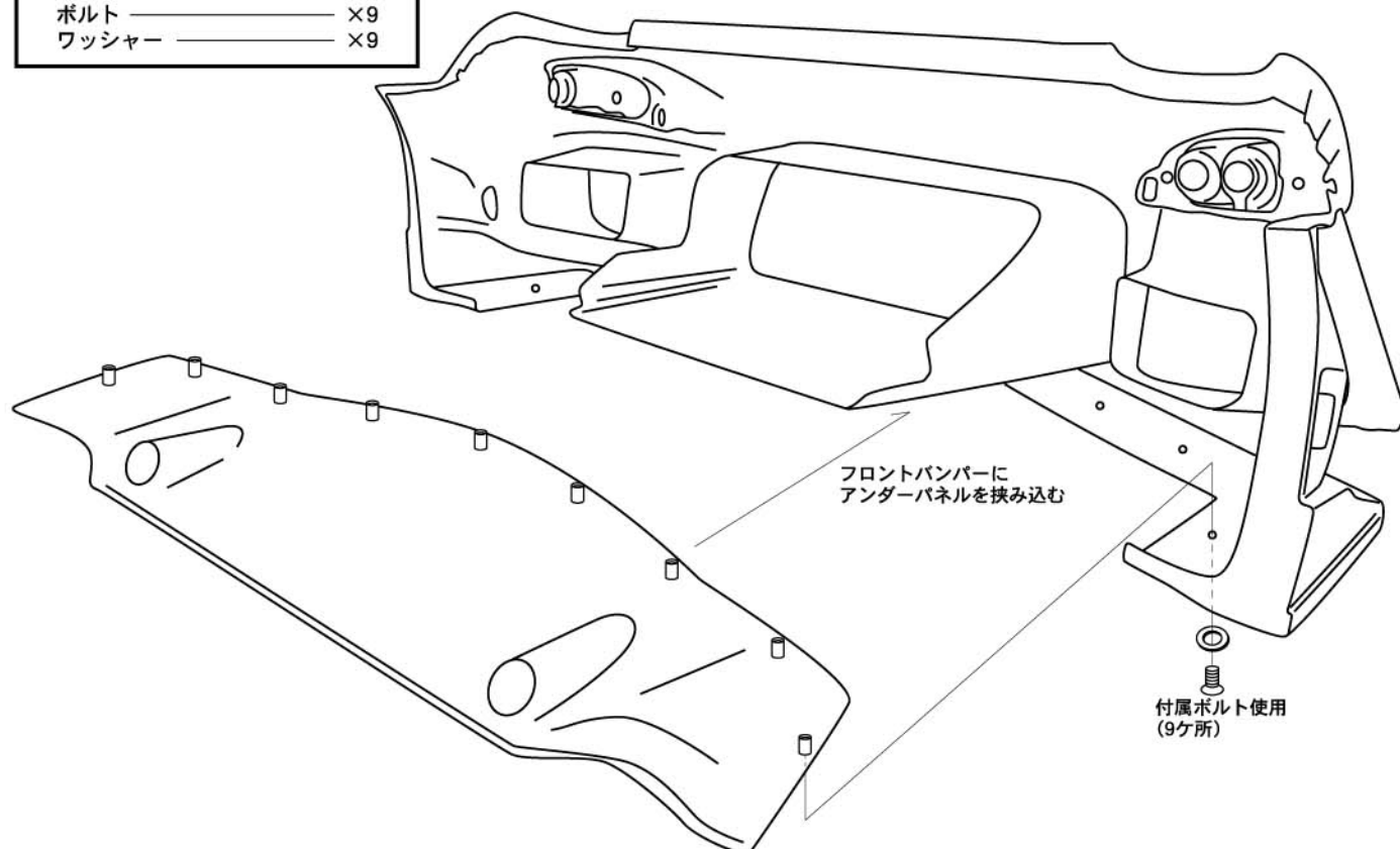
取付け図(下から見上げた図)
