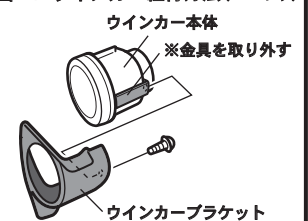
図1. ウインカー組付方法 (86のみ)
